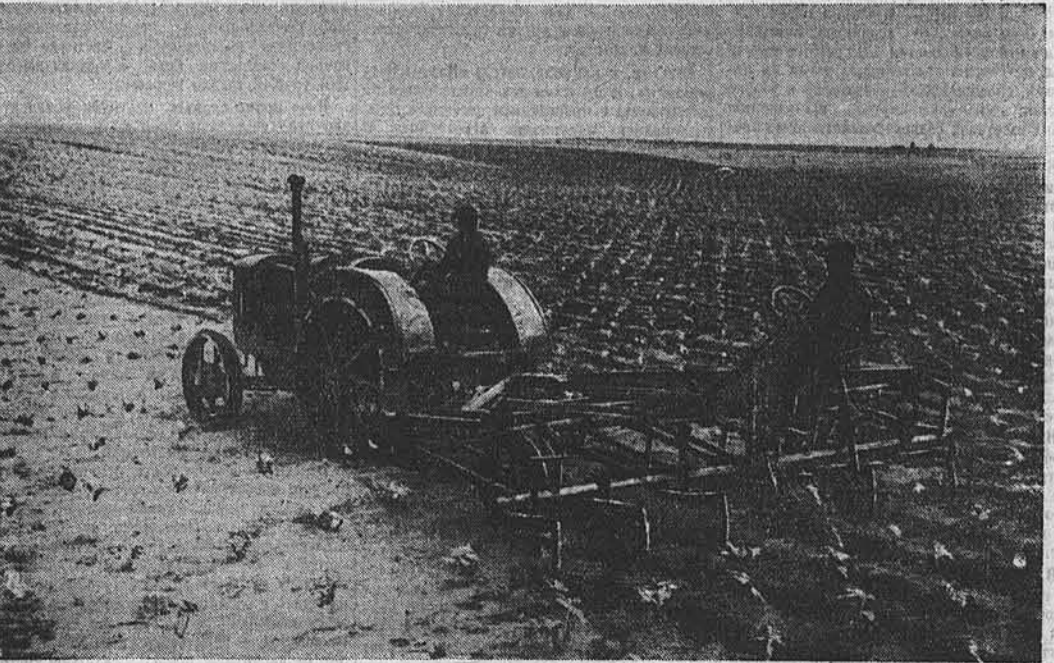
Механизаторы Ново-Егорьевской МТС и колхозники посеяли в этом году 1.160 гектаров подсолнечника и кукурузы квадратно-гнездовым способом. Сейчас они ведут уход за посевами. На снимке: тракторист Александр Осипов из тринадцатой тракторной бригады культивирует подсолнечник в колхозе имени Молотова. Фото В. Наколеса.
