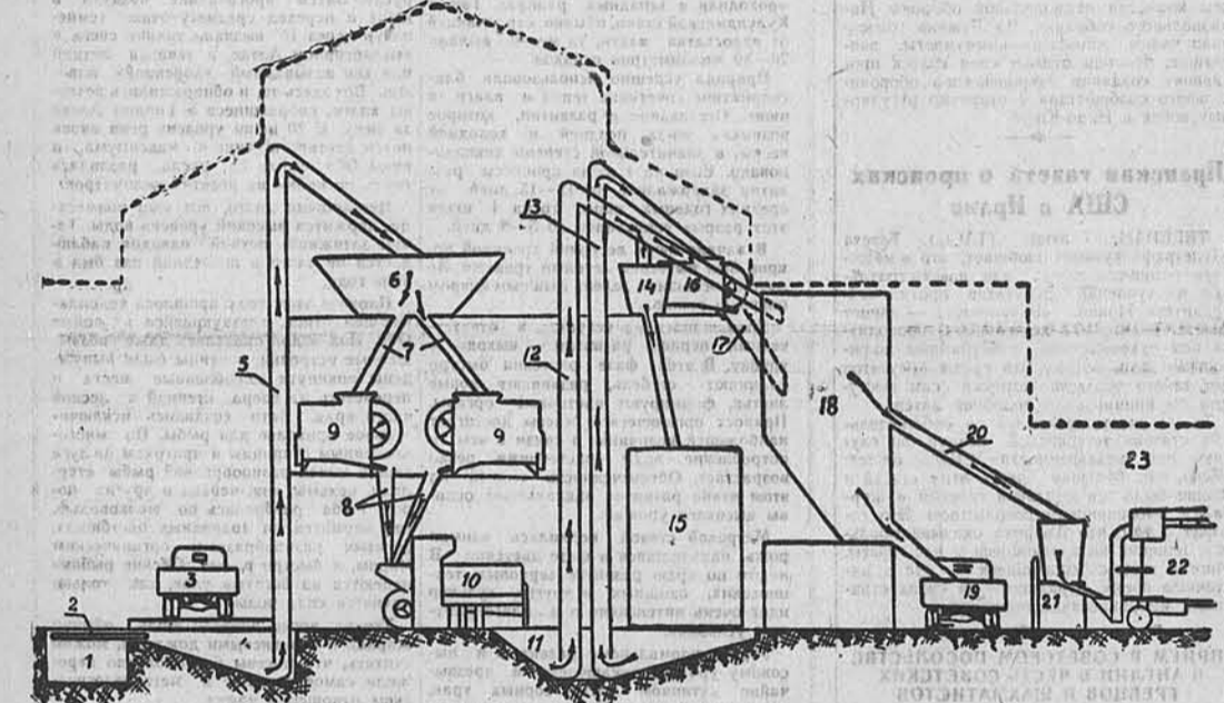
СХЕМА ЗЕРНООЧИСТИТЕЛЬНО-СУШИЛЬНОГО АГРЕГАТА ЗЕРНОСОВХОЗА ИМЕНИ 25 ЛЕТ ОКТЯБРЯ. 1-траншея ленточного транспортера, 2-ленточный транспортер, 3-автомашина под разгрузку, 4-завальная яма сырого неочищенного зерна...
