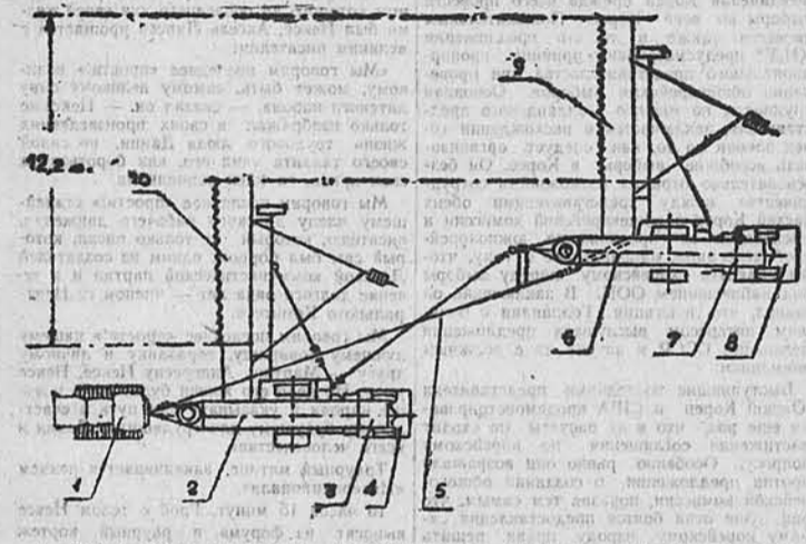
Рис. 1. Схема агрегата для заготовки силоса (1—трактор С-80, 2 и 6 — ковши «Сталинец-6», 3 и 7 — соломотранспортеры, 4 и 8 — автомашинки ЗИС-5, 5 — сцепка комбайнов, 9—10 — жатки комбайнов «Сталинец-1»).
