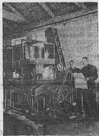
БЕЛОРУССКАЯ ССР. Завод «Гомельмаш» изготовляет нормоприготовительный комбайн «КПМ-1,5». Все процессы, начиная от загрузки исходных продуктов в комбайн и кончая выгрузкой приготовленной кормосмеси в транспортную тележку, выполняются без применения ручного труда, автоматическими. Его производительность — 1,500 килограммов кормосмеси в час. Комбайн обслуживает один человек.
