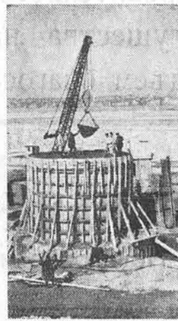
Сталинградгидрострой. Полным ходом идет подготовка к монтажу ипной подвесной дороги, которая соединит правый берег Волги с островом Песчаным. Сейчас на острове ведется бетонирование опор.
