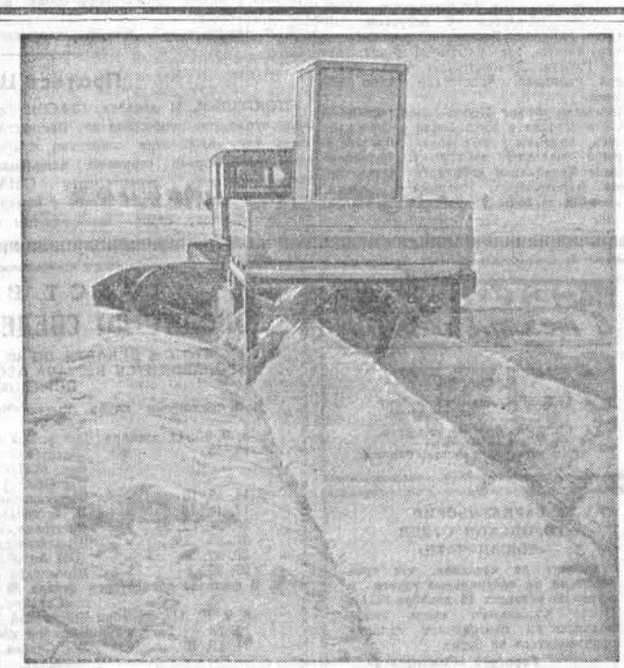
Снеговый пресс конструкции Б. Е. Сквородникова за работой. Фото Н. Калинин.
