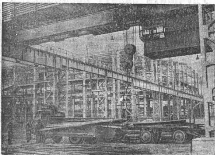
ПОЛЬША. Близ Кракова строится по советскому проекту гигант польской промышленности — металлургический комбинат Нова Гута. Один за другим вступают в строй промышленные объекты. НА СНИМКЕ: смонтированный межколевой транспортер советской конструкции. Фото Польского агентства печати.
