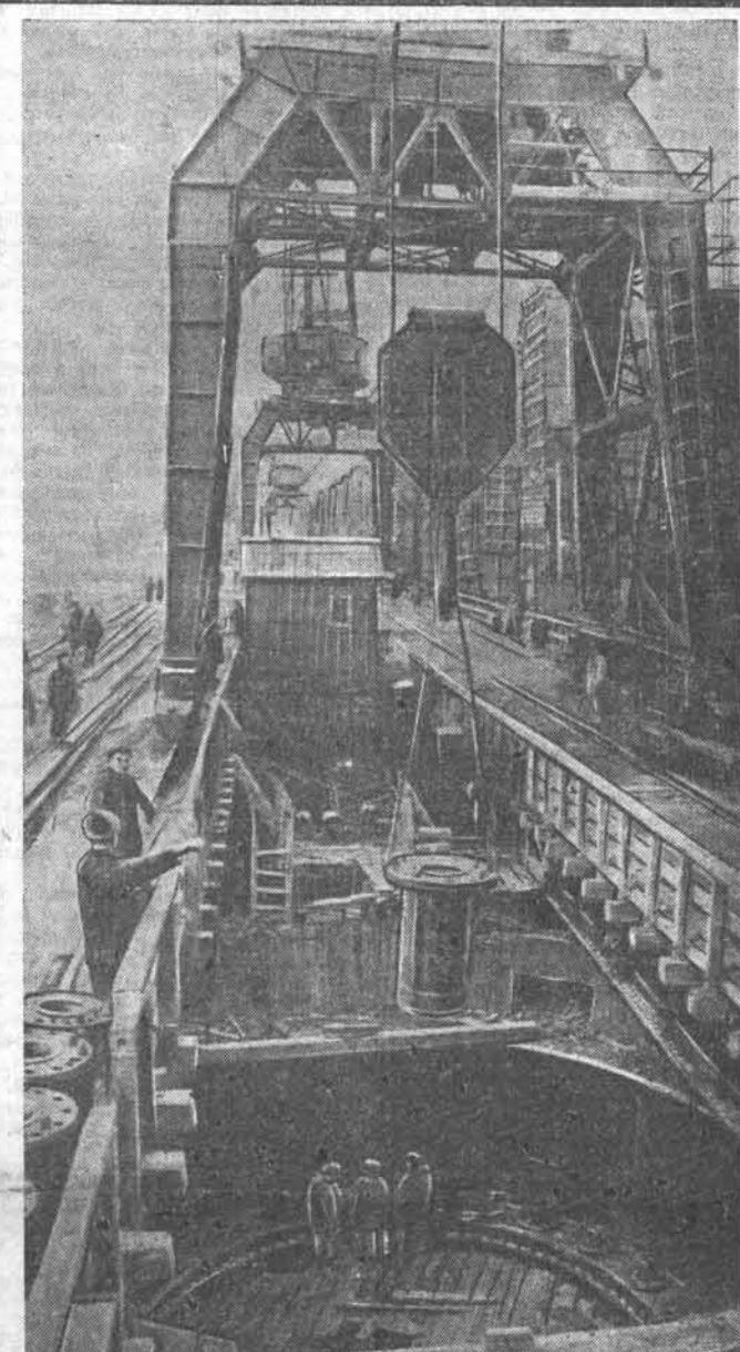
ВОЛГОДОНСТРОЙ. На строительстве Цимлянской гидроэлектростанции идет монтаж турбин. НА СНИМКЕ: сборка опорного кольца, на которое будет установлена одна из турбин Цимлянской гидроэлектростанции. Фото С. Кривонизицкого. (Фотохроника ТАСС)
