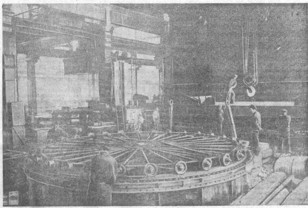
ЛЕНИНГРАД. Коллектив завода под'емно-транспортного оборудования имени С. М. Кирова выполняет почетные заказы для строек коммунизма. НА СНИМКЕ: сборка 10-тонного порталного крана для строительства Волго-Донского канала. Фото А. Михайлова. (Фотохроника ТАСС).
