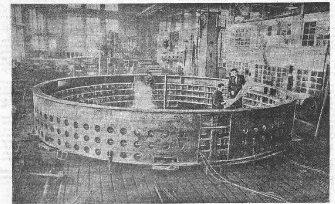
ВО ИМЯ МИРА. В цехах Ленинградского завода «Электросиль» имени С. М. Кирова огромный трудовой подвиг. С величайшим воодушевлением коллектив завода выполняет почетные заказы для великих строек коммунизма. На снимке: сборка гидрогенератора для Цимлянкой ГЭС. Фото А. Михайлова. (Фотохроника ТАСС).
