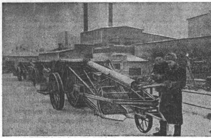
Рязанский завод сельскохозяйственного машиностроения «Рязсельмаш» производит серийный выпуск комбайнов КОК-2 для уборки картофеля. НА СНИМКЕ: контролер отдела технического контроля В. М. Николаев (слева) принимает от мастера сборочного цеха В. Г. Цепулина новые комбайны КОК-2. Фото Н. Стрелюва (Фотохроника ТАСС).
