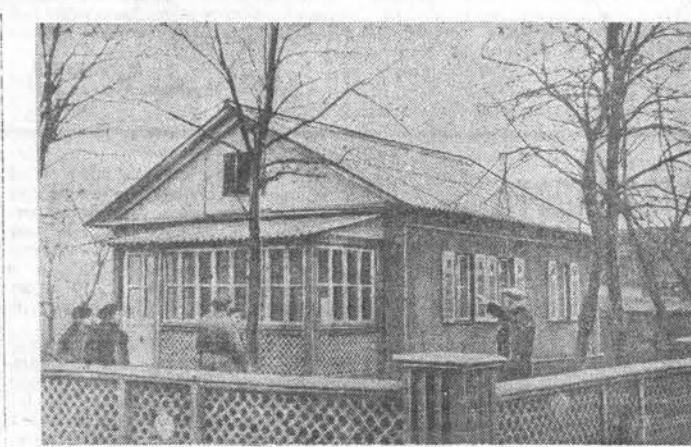
Украинская ССР. В Макеевке, в посёлке завода имени Кирова, трест «Макстрой» построил первый сборный жилой дом из железобетонных деталей. В нём три комнаты и кухня-столовая, жилая площадь — 46 квадратных метров. Все части дома изготовлялись в цехах и мастерских треста «Макстрой», затем были завезены на площадку и смонтированы при помощи автокрана на заранее подготовленных фундаментах. Изготовление деталей дома в заводских условиях позволило значительно индустриализировать строительство. НА СНИМКЕ: внешний вид сборного железобетонного жилого дома. Фото С. Гендельмана. (Фотохроника ТАСС).
