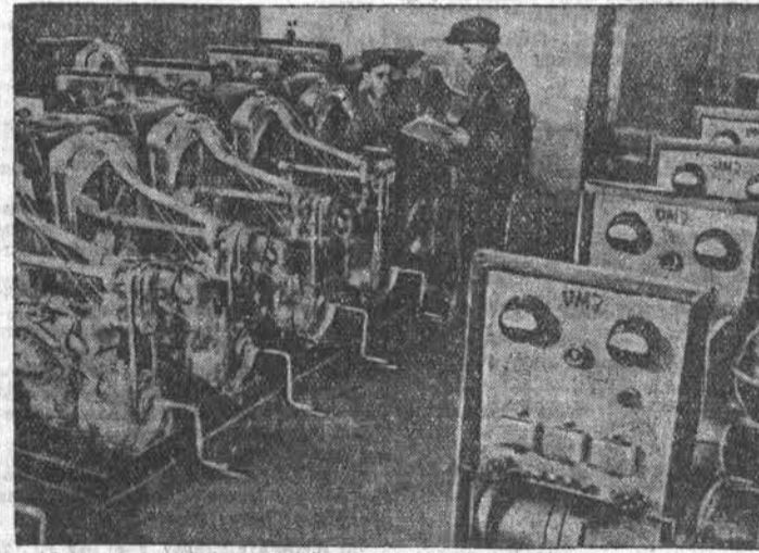
Латвийская ССР. Рижский механический завод освоил выпуск передовых электростанций, предназначенных для питания электроламп и других силовых электростанций на лесозаготовках. Большое количество этих электростанций отправлено в лесопромышленные районы нашей страны. С переходом на поточный метод сборки выпуск электростанций в 1950 году значительно увеличился. НА СНИМКЕ: подготовка к отпарке электростанций. Фото Б. Федосеева. (Фотохроника ТАСС).
