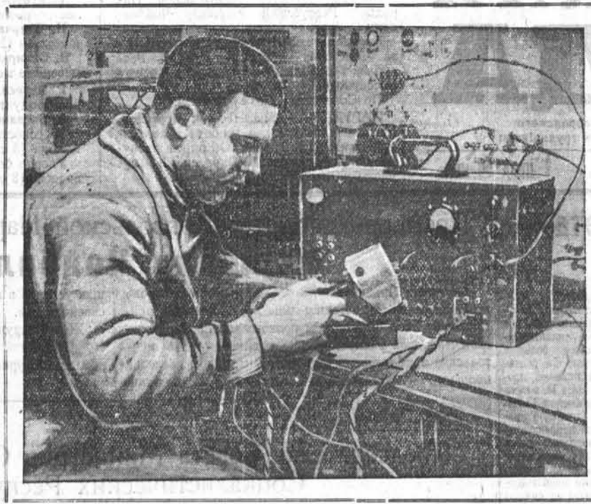
На Барнаульском ордена Трудового Знамени вагоноремонтном заводе в последнее время стал наиболее широко применяться электроскоровый метод обработки инструмента. Особенно большие успехи в этом отношении достигнуты в прессовом отделении кузнечного цеха. Повышение стойкости инструмента позволило значительно увеличить выпуск продукции и сократить расход инструмента. НА СНИМКЕ: лаборант Е. И. ТИТОВ за процессом электрошлифования резцов. Фото Н. Суворовской.
