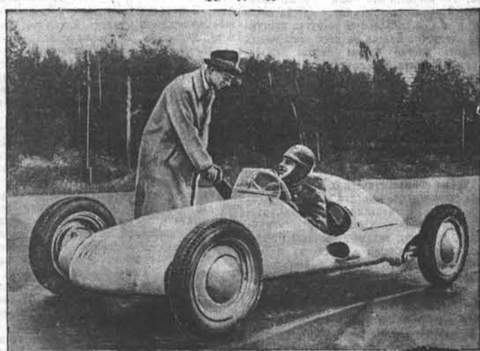
Под Москвой были проведены спортивные испытания нового дорожно-гоночного автомобиля «Салют-М» конструкции инженера М. Дерковского. Испытание было организовано Комитетом по делам физкультуры и спорта при Совете Министров РСФСР.
