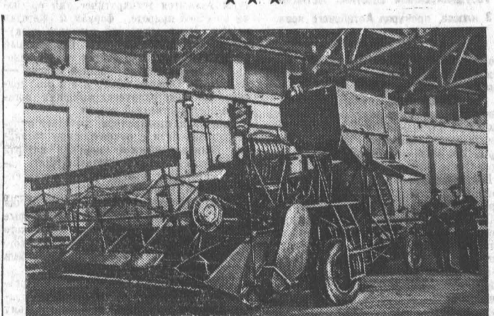
В Казани, на заводе самоходных комбайнов выпущен первый опытный образец самоходного комбайна «С-4». Идет подготовка к серийному выпуску машины. Коллектив предприятия обязался к 30-й годовщине Октября выпустить 300 комбайнов «С-4». НА СНИМКЕ: первый образец самоходного комбайна в цехе завода. (Фотохроника ТАСС).
