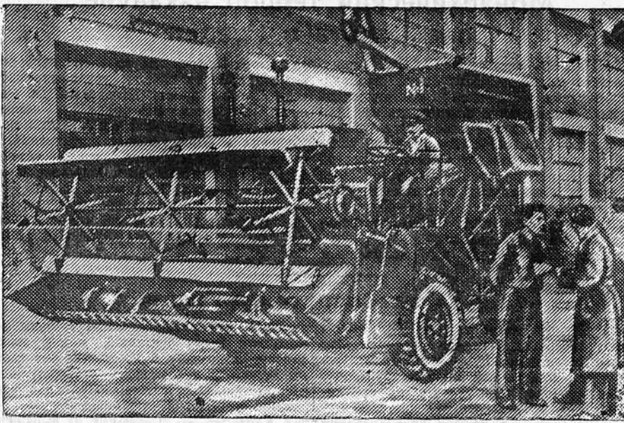
ПЕРВЫЙ СОВЕТСКИЙ САМОХОДНЫЙ КОМБАЙН. На Московском заводе имени Владимира Ильича построен первый советский самоходный комбайн „ЖМС-4,0“. Он изготовлен по проекту, разработанному группой конструкторов Всесоюзного научно-исследовательского института сельскохозяйственного машиностроения под руководством доктора технических наук М. А. ПУСТЫГИНА и инженера И. С. ИВАНОВА.
