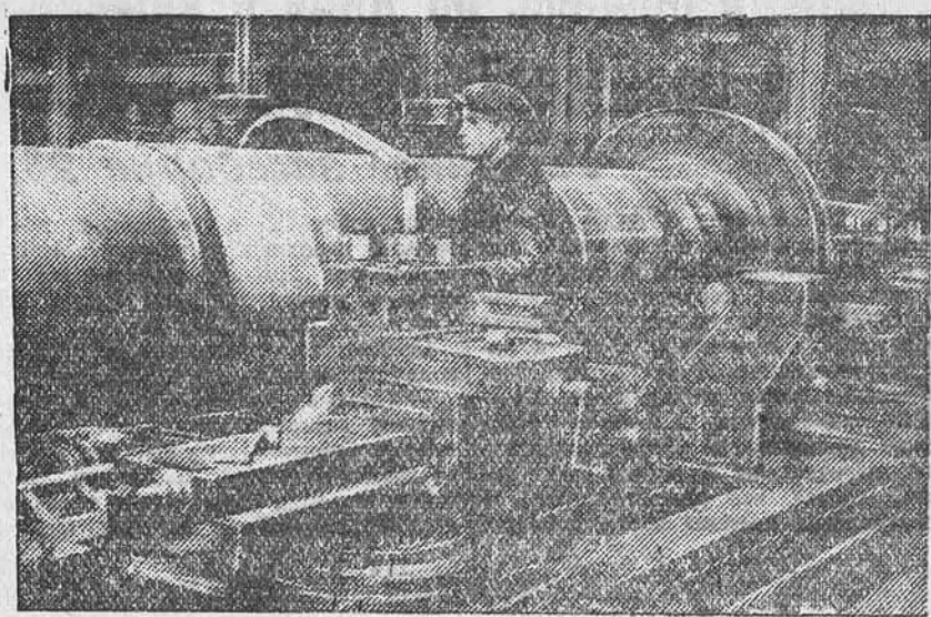
Ленинградский государственный ордена Ленина и Трудового Красного Знамени завод «Электросила» имени С. М. Кирова изготовляет гидрогенератор для Нижне-Свирской гидроэлектростанции (мощность в 30 тысяч киловатт). НА СНИМКЕ: стахановец завода токарь С. Д. БОЙЧЕНКО за обточкой 10-метрового вала гидрогенератора. Фото Н. Караева (Фотохроика ТАСС).
