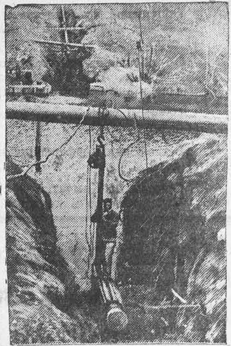
На строительстве газопровода Саратов—Москва. Экспедиция подводных работ, где начальником техник-лейтенант В. И. Пудан, прокладывает газопровод по дну реки Пахра (Московская область). НА СНИМКЕ: момент опускания труб газопровода. Фото Д. Минсера. (Фотохроника ТАСС).
