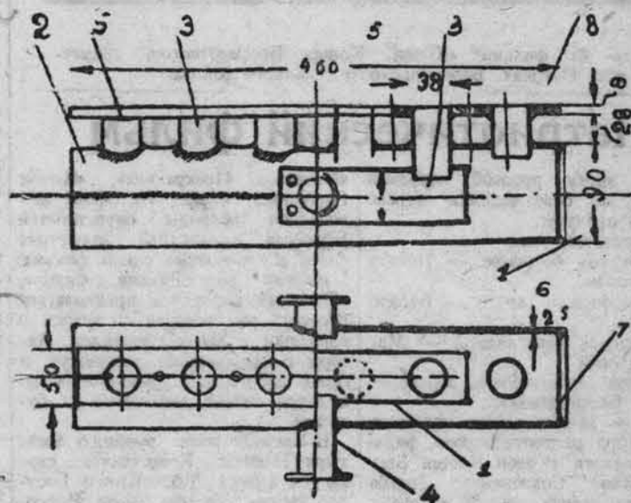
Сварной коллектор мотора комбайна ГАЗ-НАТИ для работы на керосине.
