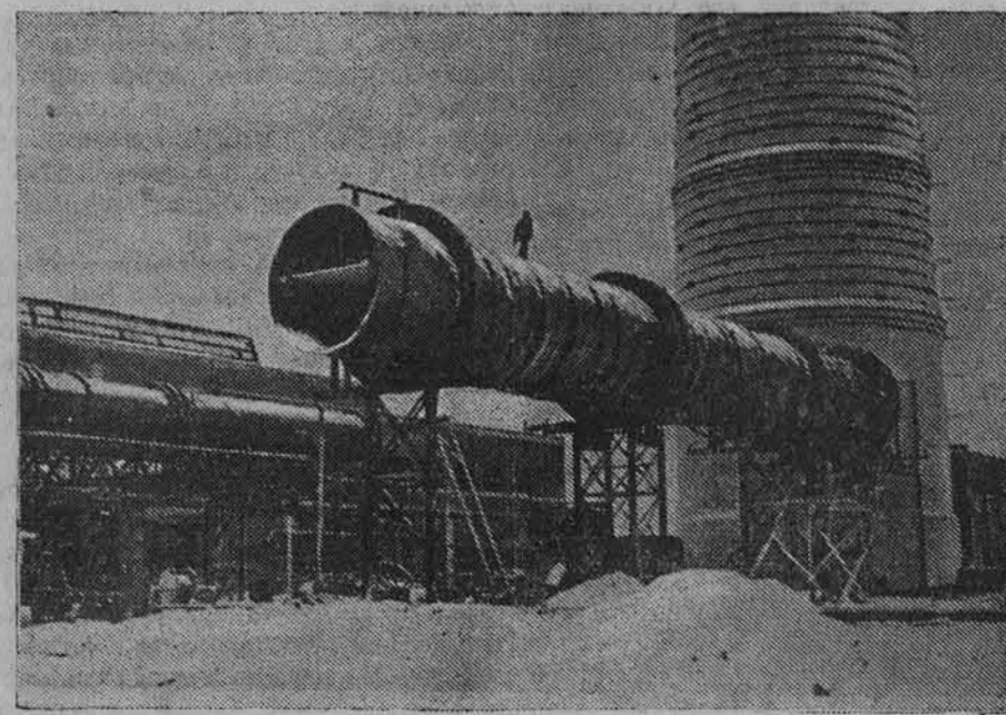
На строительстве Среднеуральского металлургического завода. НА СНИМКЕ: монтаж газопровода. Фото В. Носкова. (Фото-кино ТАСС).
