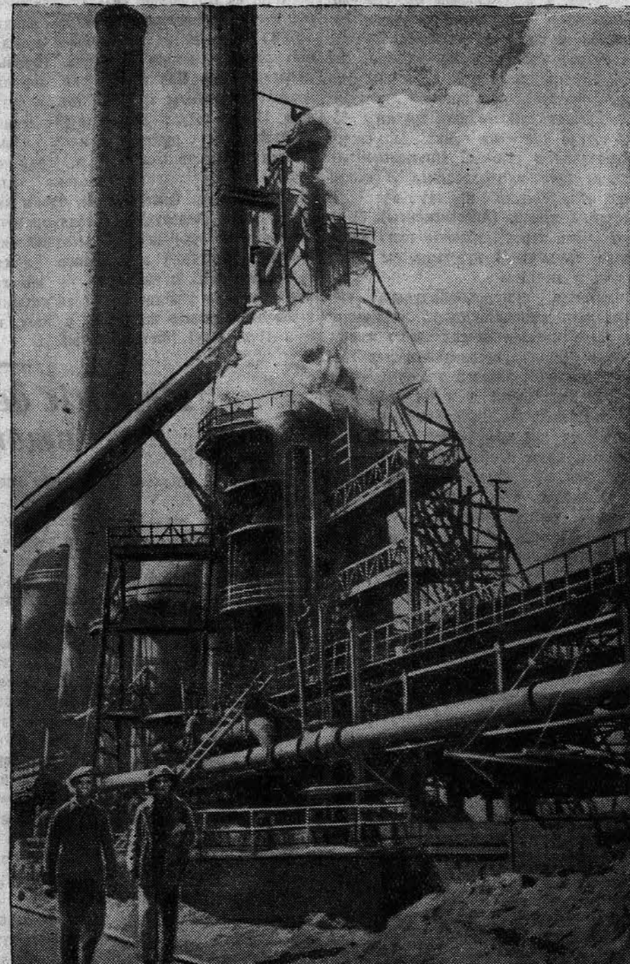
Доменная печь № 2 Днепродзержинского завода металлургического оборудования переоборудуемая на кислородное дутье. Фотохроника ТАСС.
