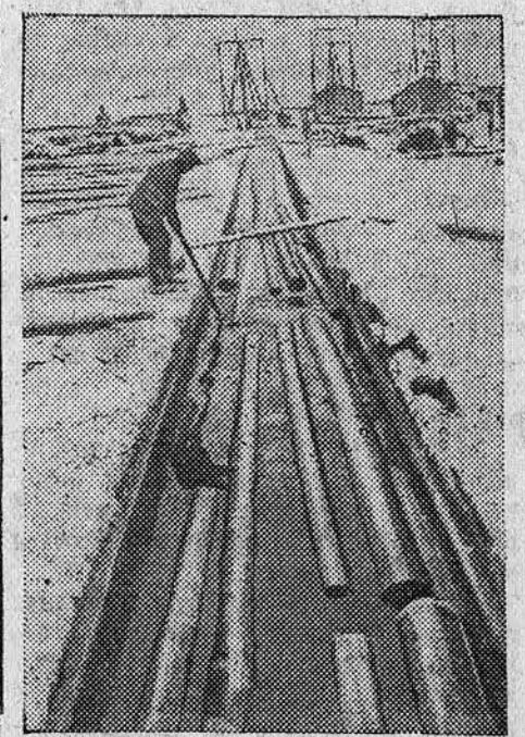
Архангельский лесопильный завод имени Молотова — крупнейший лесопильный завод в СССР. Он имеет 24 лесопильных рамы и выпускает 4000 кубометров досок в день. Большинство процессов на заводе механизировано. НА СНИМКЕ: транспортировка леса со склада на лесопильные рамы системы проточных бассейнов (или лотков, с подогревой водой. Этот метод, впервые примененный здесь, дал заводу большую экономию, увеличил производительность завода на 50 процентов. Фото Б. Дорофеева (Фотохроника ТАСС)
