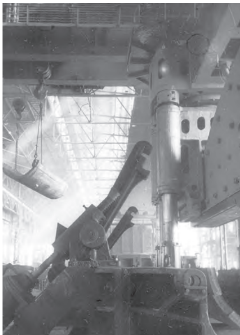
Барнаулский котельный завод. Пресс «механическая рука». Фото Н. Калинина. 1966 г. ГААК. Фотодокументы. Оп. 2. Д. 0-2364.
