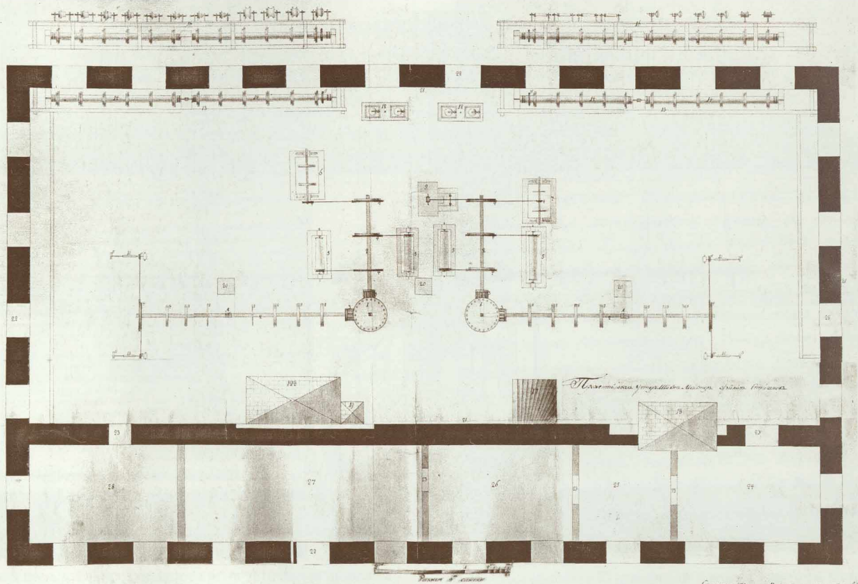
№ 13 Проектный план шлифовальной фабрики при Кольванском заводе, составленный унтер-шихтмейстером Стрижковым. [Конец XVIII в.] ЦХАФ АК. Ф. 50. Оп. 19. Д. 216, 224, 225. Копия.
