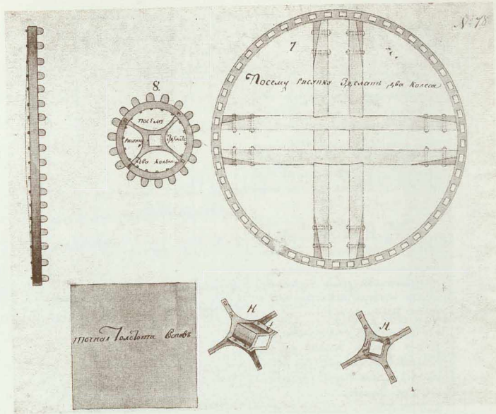
№ 7 Рисунки шлифовальных колес. 1792 г. ЦХАФ АК. Ф. 50. Оп. 19. Д. 222. Подлинник.
