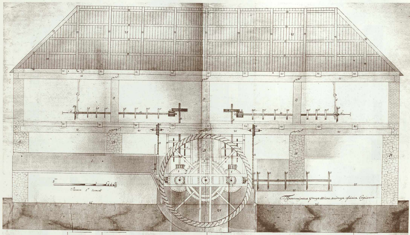
№ 12 Проектный план шлифовальной фабрики при Колыванском заводе, составленный унтер-шихтмейстером Стрижковым. [Конец XVIII в.] ЦХАФ АК. Ф. 50. Оп. 19. Д. 216, 224, 225. Копия.
