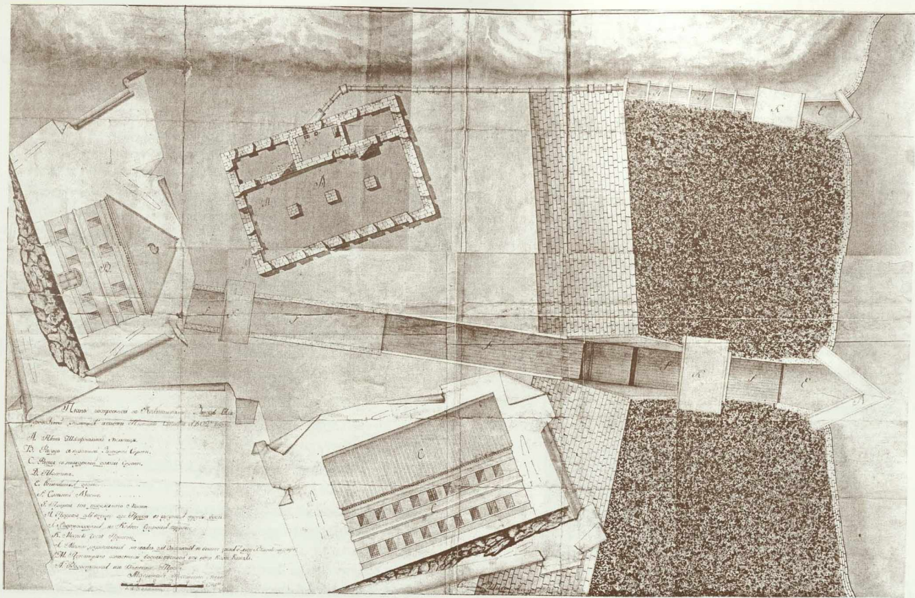
№ 14 План построенной в Колыванском заводе шлифовальной мельницы и части плотины. 1802 г. ЦХАФ АК. Ф. 50. Оп. 19. Д. 228. Подлинник.
